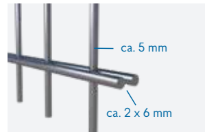
Typ 6/5/6
