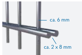
Typ 8/6/8
